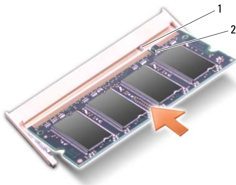
1 languette 2 encoche
