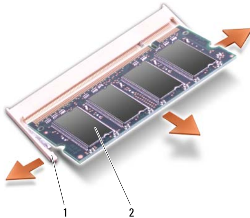
1 clips de fixation (2) 2 module de mémoire (DIMM 1)
