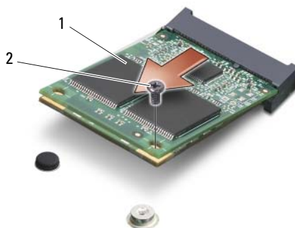
1 carte FCM 2 vis M2 x 3 mm
